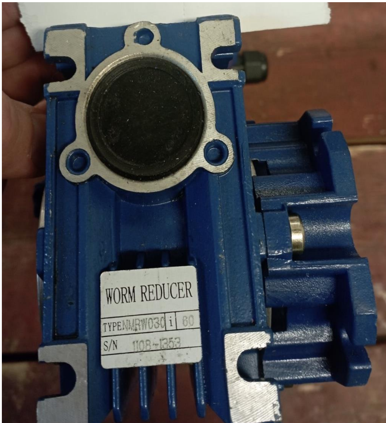
Мотор редуктор NMRV030-60-23,3-0,18
